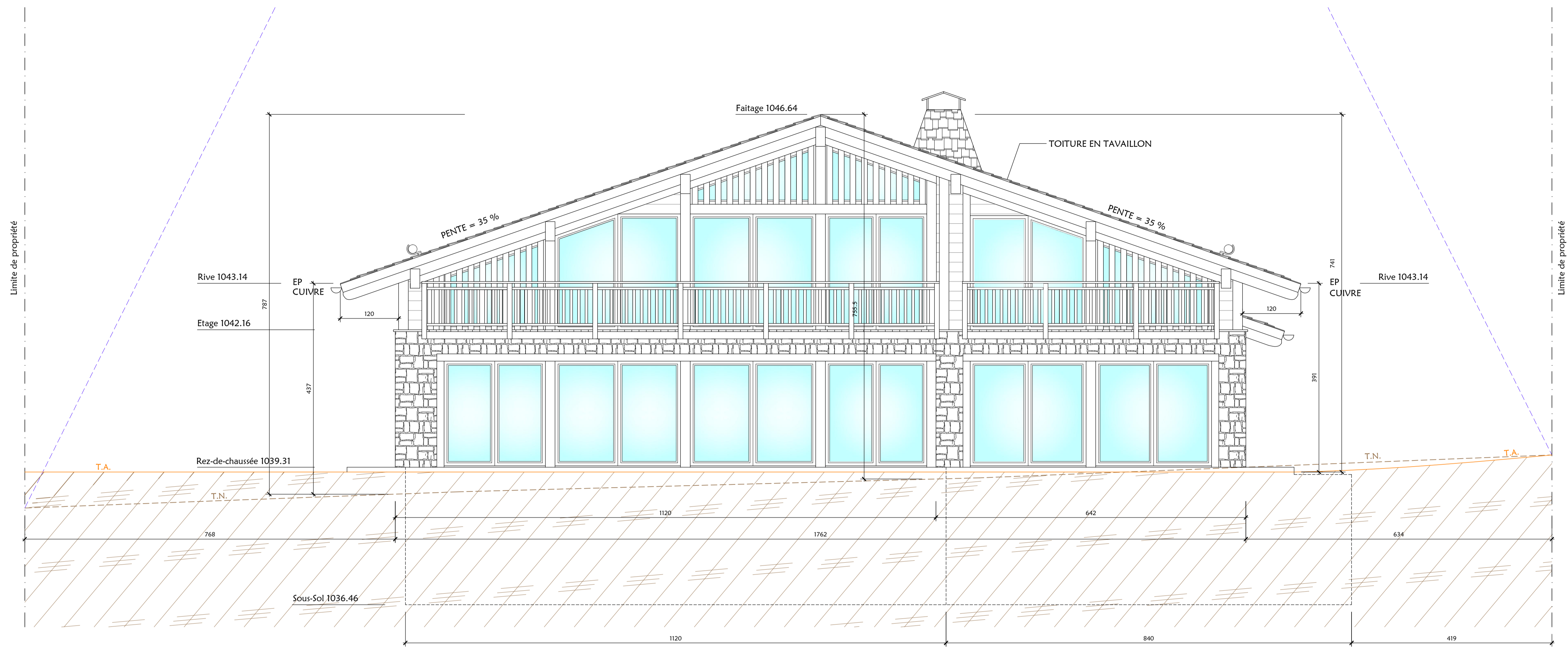
PLAN DE FACADES SUD-OUEST
