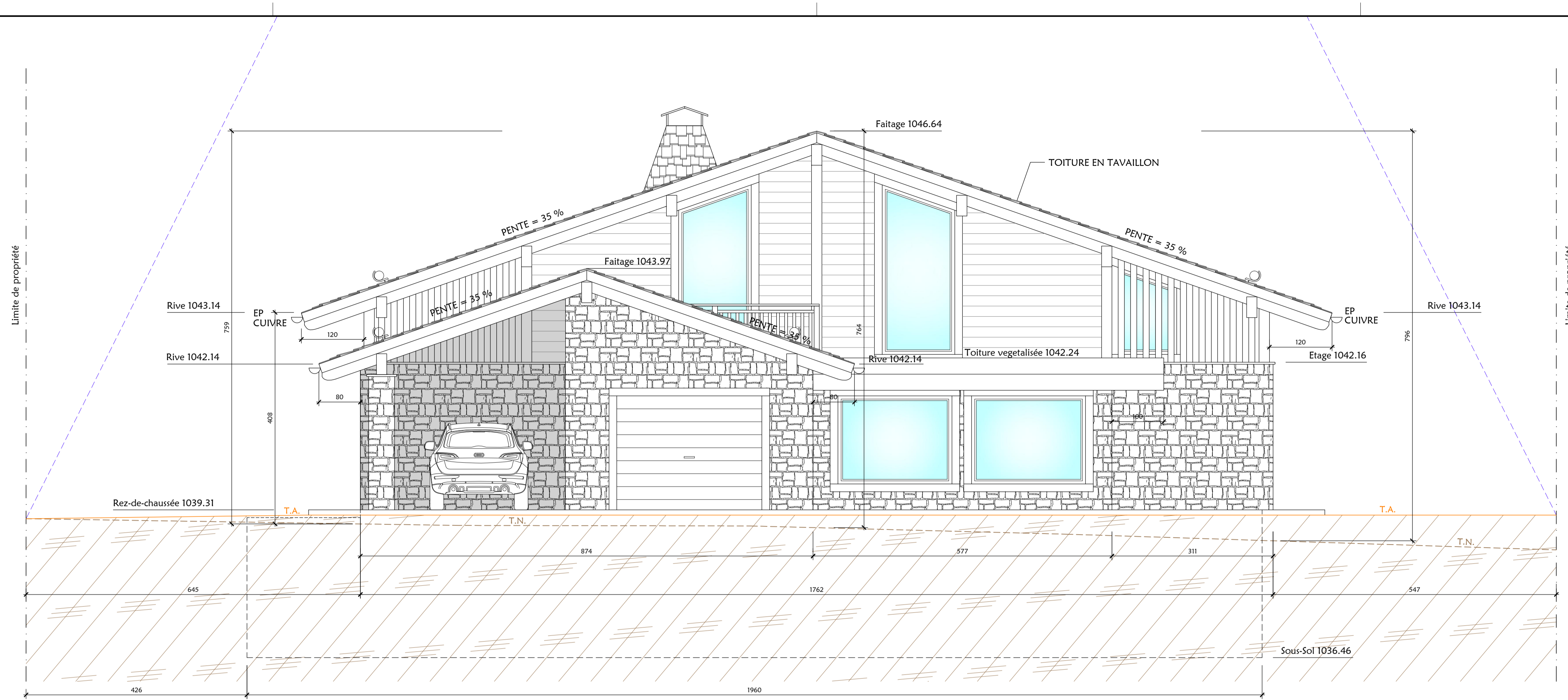
PLAN DE FACADES SUD-EST
